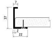
výkres k úchytkce QE33 (mm)
