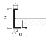
výkres k úchytkce E34 (mm)
