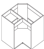
KTS007-B - korpus spodní rohový dřezový zalomený, vlys vodorovný
