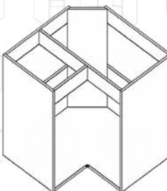
KTS007-B - korpus spodní rohový dřezový zalomený, vlys vodorovný
