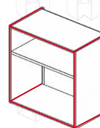
KORPUSY HORNÍ A VYSOKÉ všechny čtyři hrany
