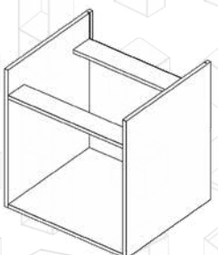
KTS005 - korpus spodní varná deska
