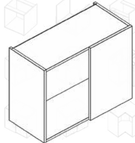
KTH003-P - korpus horní rohový - rovný pravý
